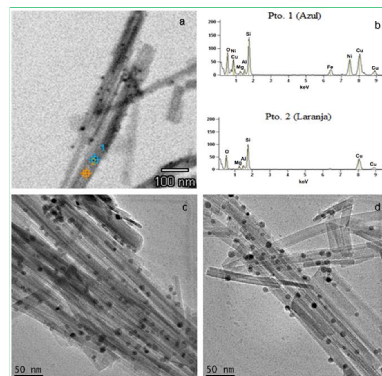
Micrografias (MET) e microanálise (EDS) dos Nanotubos Ativados com nanopartículas de Ni incorporado (H 2 /Ar) (PA-Ni550r).
