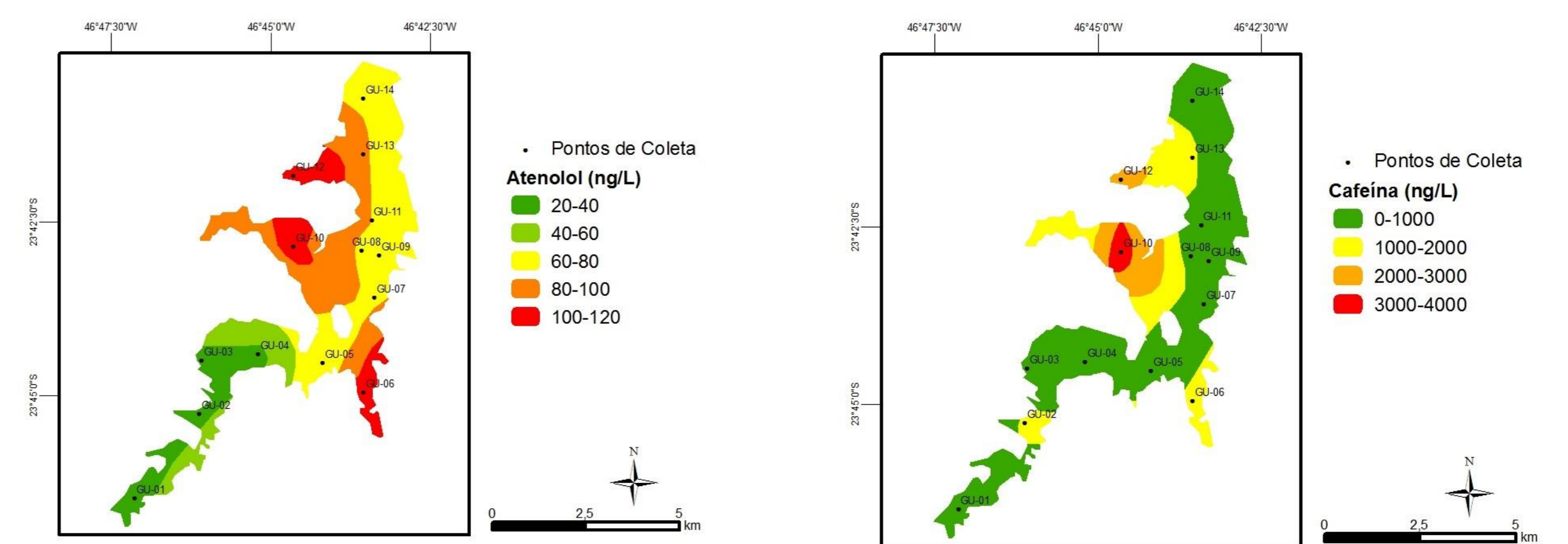
Distribuição do fármaco atenolol e da cafeína nas águas do Reservatório do Guarapiranga
